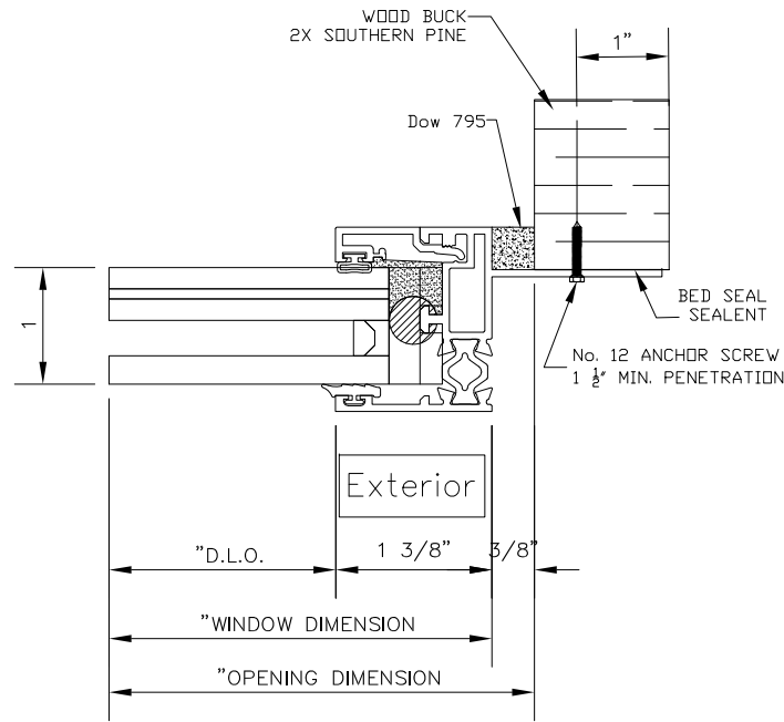
E JAMB Frame Depth: 1.625
